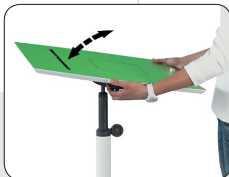
Neigungsverstellung der Pultplatte: 0° bis 70° in sieben Stufen
